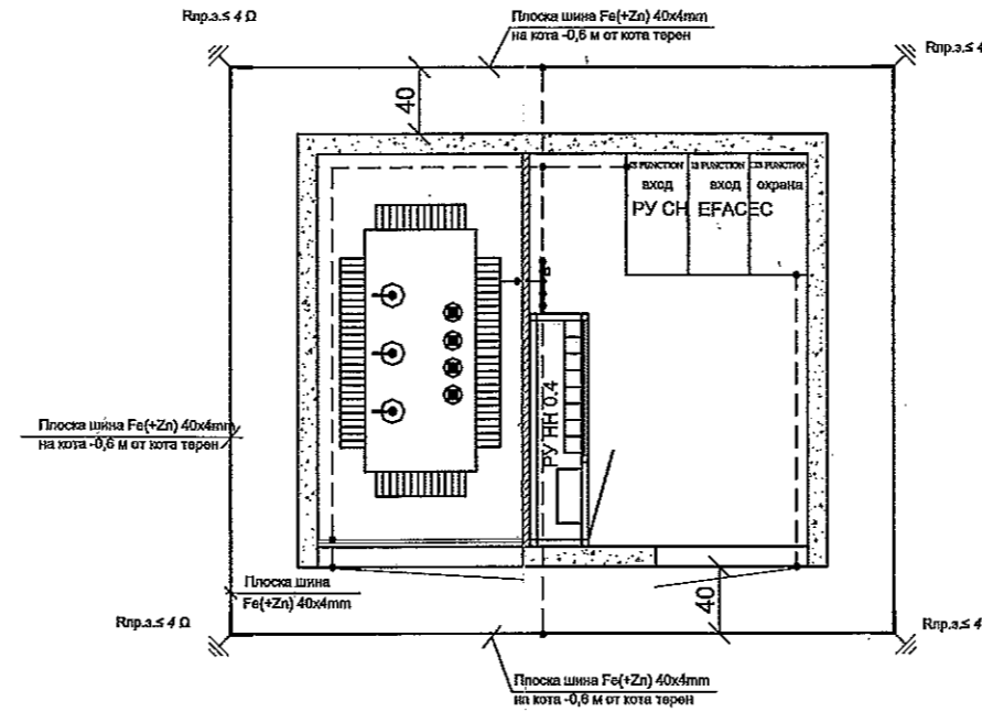
ЗАЗЕМЛЕНИЕ
