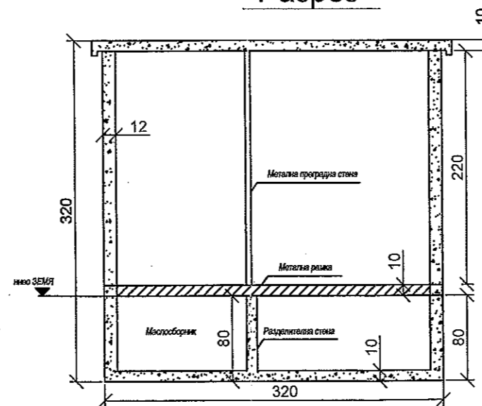
Разрез
