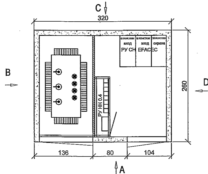
КОМПАНОВКА
